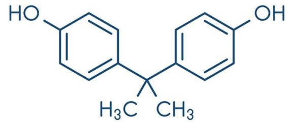
bisphenol A
